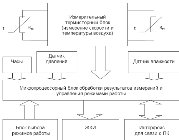
Рис. 1 Блок схема Измерителя
